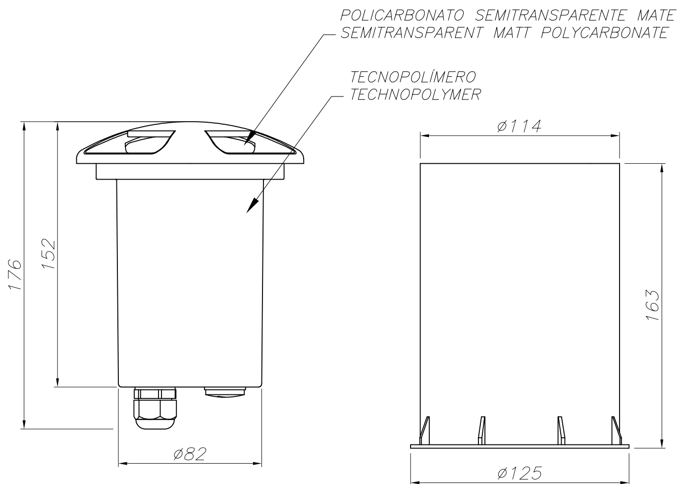
CAJA DE EMPOTRAR FLUSH FITTING BOX
